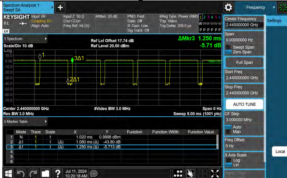
NTNV-BLE_2M-Ant1-2440
