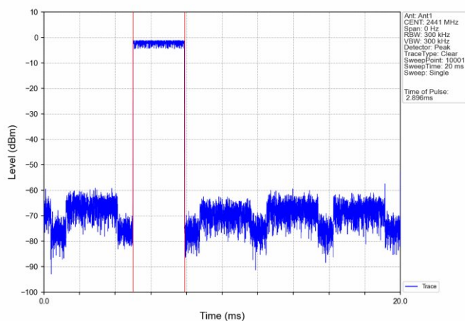
GFSK_DH5_HOPP_Ant1_NTNV
