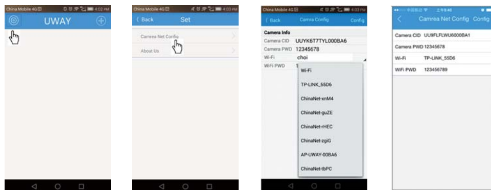
Android
