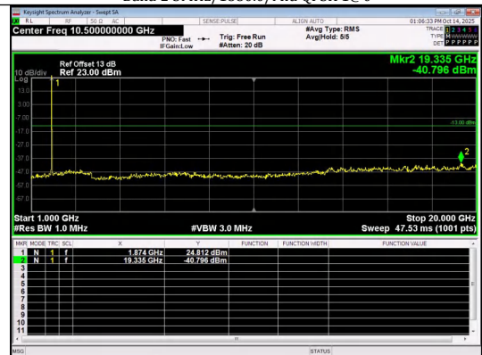
1000.0MHz-20000.0MHz Band 2 5MHz/1880.0/Mid 16QAM 1@0
