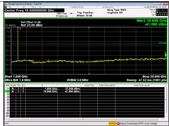
1000.0MHz-20000.0MHz Band 2 5MHz/1852.5/Low QPSK 1@0
