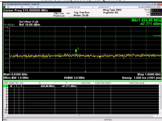
30.0MHz-1000.0MHz Band 2 5MHz/1880.0/Mid 16QAM 1@0
