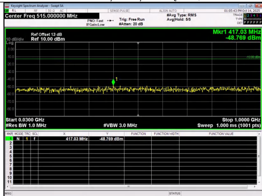
30.0MHz-1000.0MHz Band 2 5MHz/1880.0/Mid QPSK 1@0
