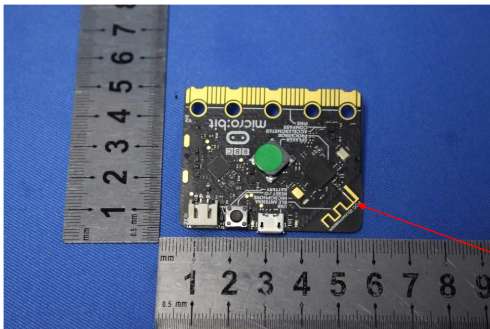
BLE antenna
