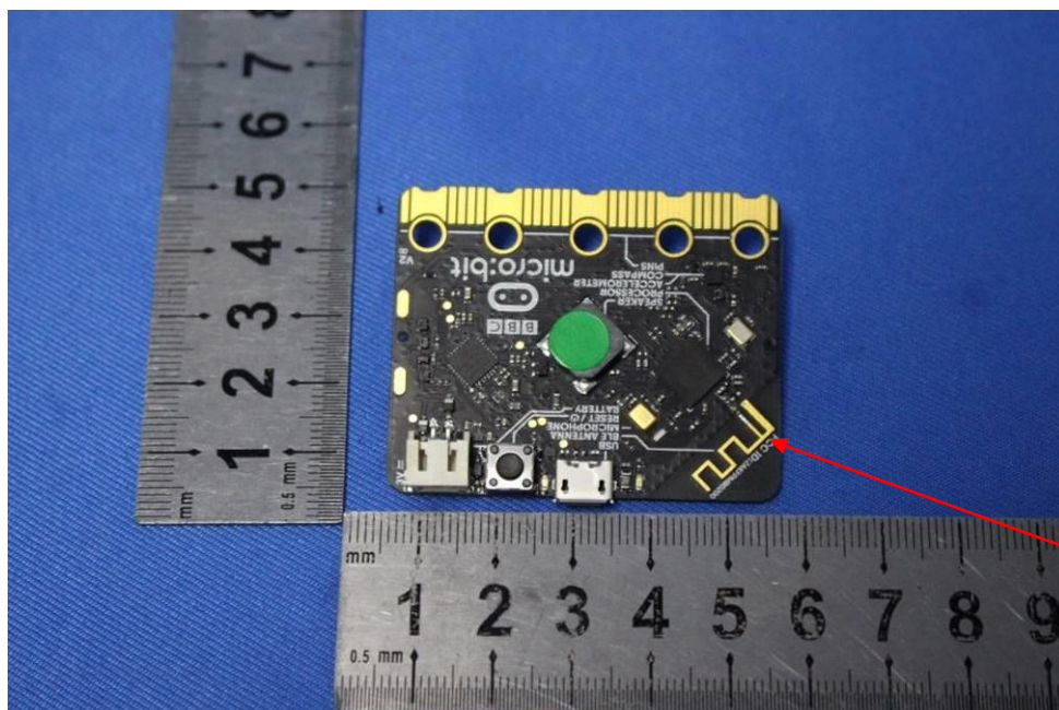
BLE antenna
