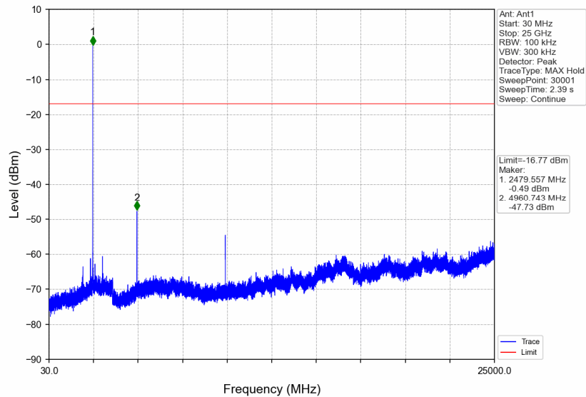
2M_HCH_2480MHz_DataRate=_Ant1_NTNV
