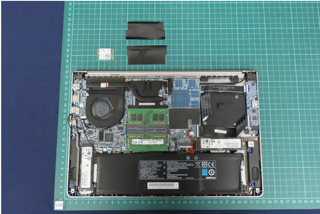
(10) EUT Photo
