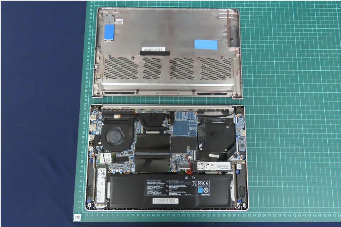
(8) EUT Photo
