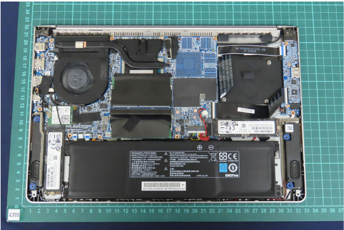
(9) EUT Photo
