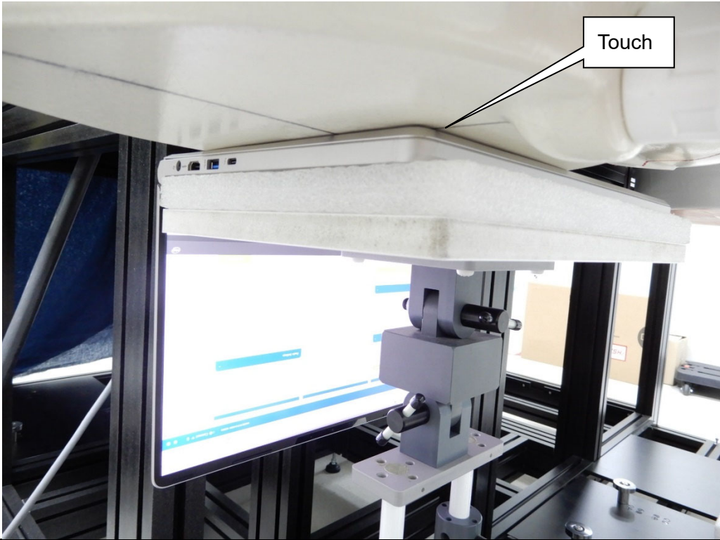
EUT Bottom_Aux
