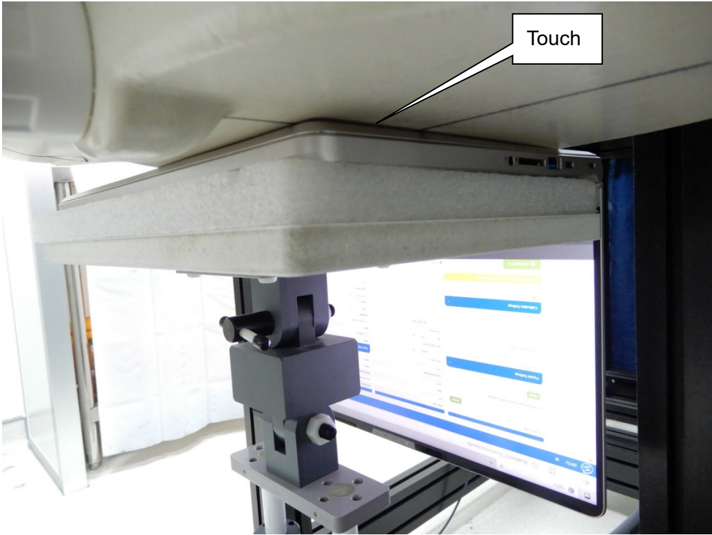
EUT Bottom_Main
