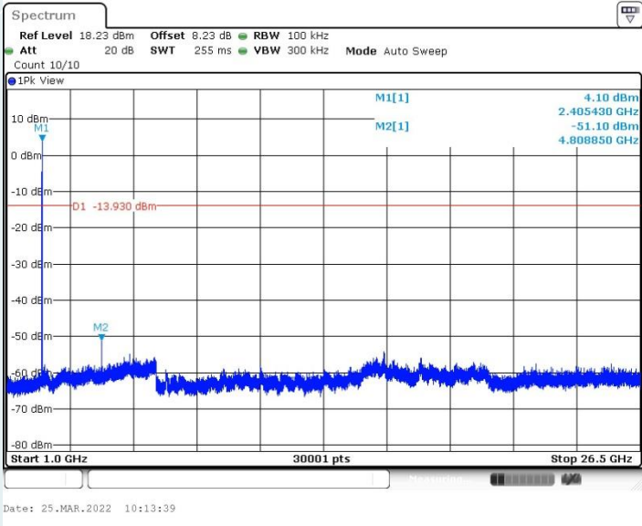
Zigbee_2405MHz_1000~26500MHz
