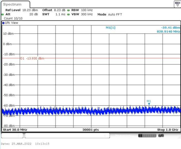
Zigbee_2405MHz_30~1000MHz
