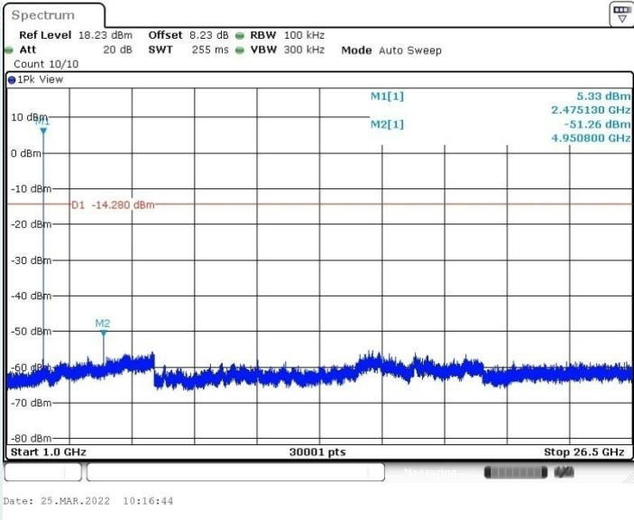
Zigbee_2475MHz_1000~26500MHz
