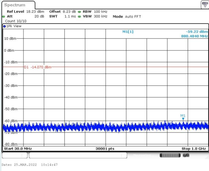
Zigbee_2440MHz_30~1000MHz
