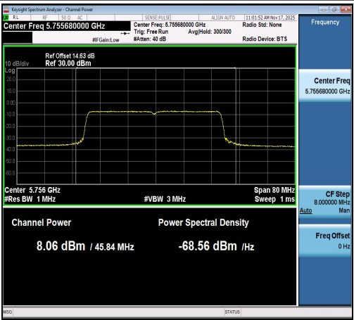
11AX40ISO-Ant1-5755-PASS
