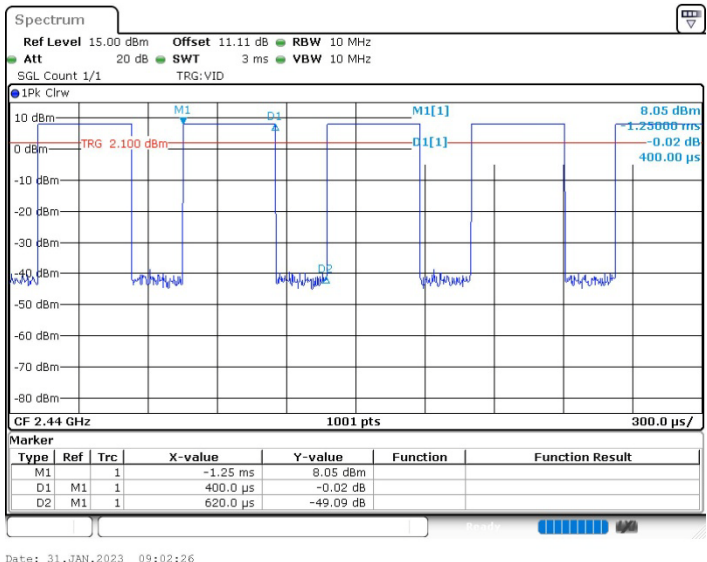
BLE_2M_2440MHz
