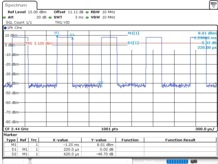
BLE_2M_2440MHz
