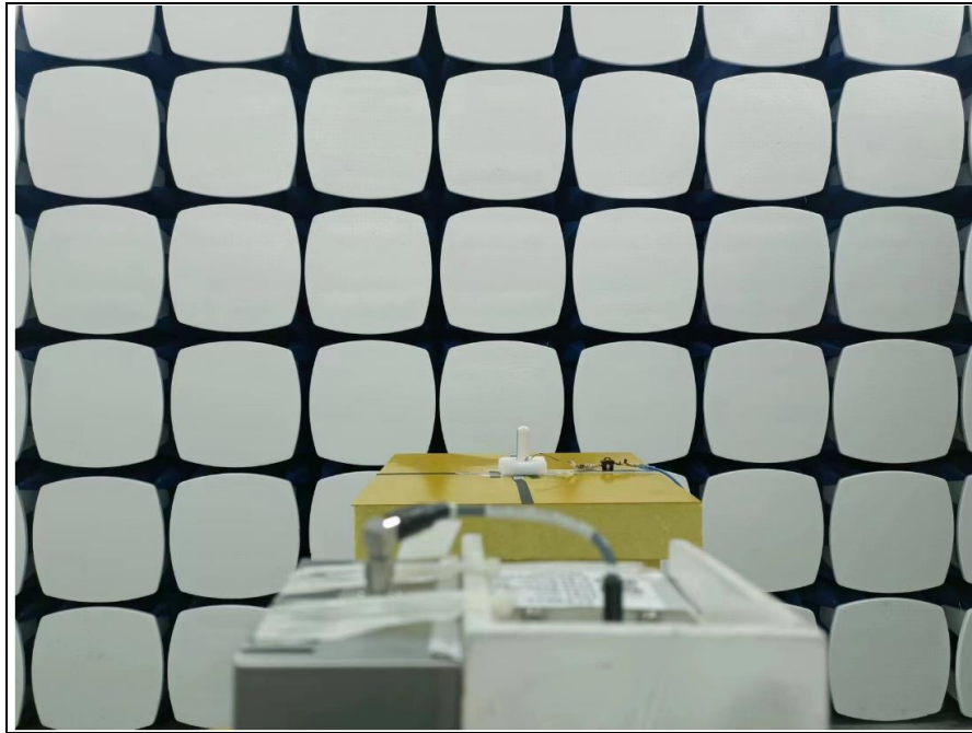
18GHz-26.5GHz(FCC&IC)
