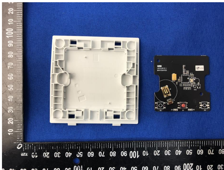
EUT UNCOVER VIEW 4 (WXKG03LM)
