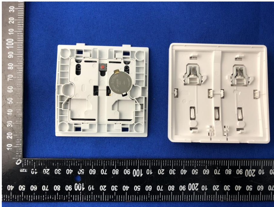
EUT UNCOVER VIEW 1 (WXKG03LM)
