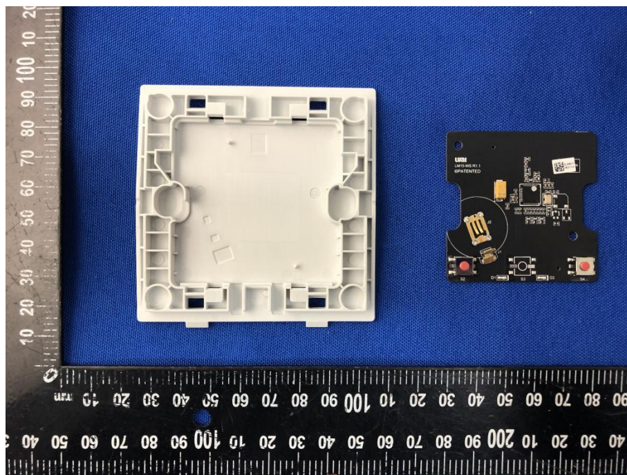
EUT UNCOVER VIEW 4 (WXKG02LM)
