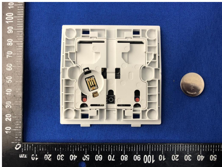
EUT UNCOVER VIEW 2 (WXKG02LM)
