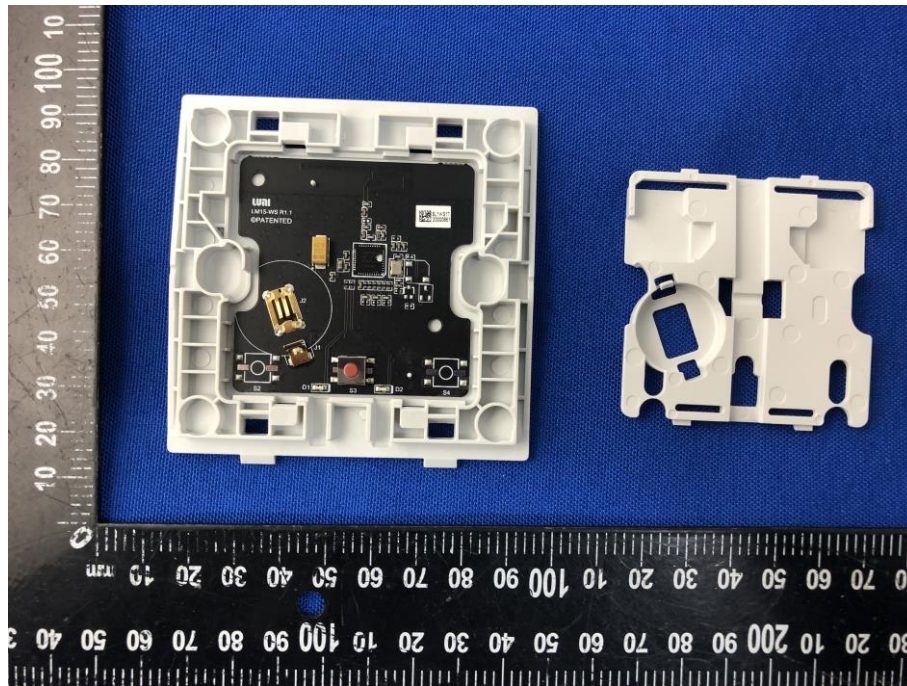
EUT UNCOVER VIEW 3 (WXKG03LM)
