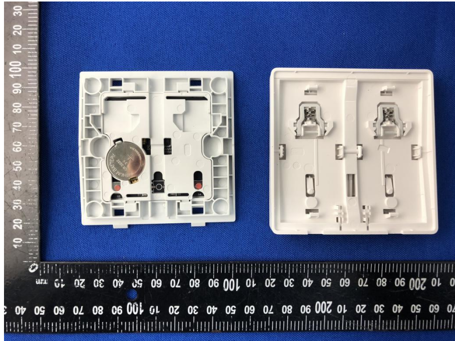
EUT UNCOVER VIEW 1 (WXKG02LM)
