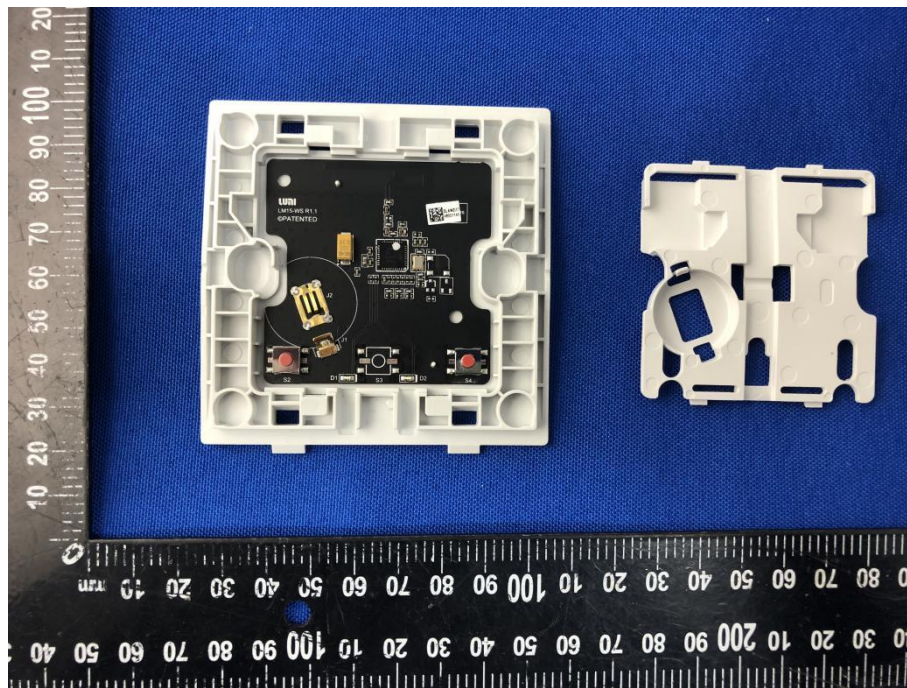
EUT UNCOVER VIEW 3 (WXKG02LM)
