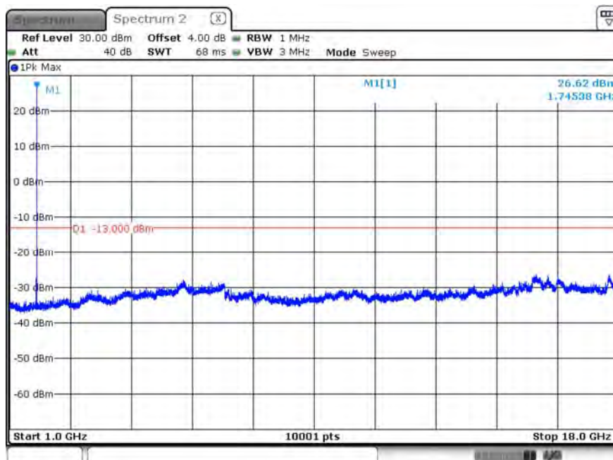
B66_CH132322_1.4M_1RB2_QPSK_Above 1G
