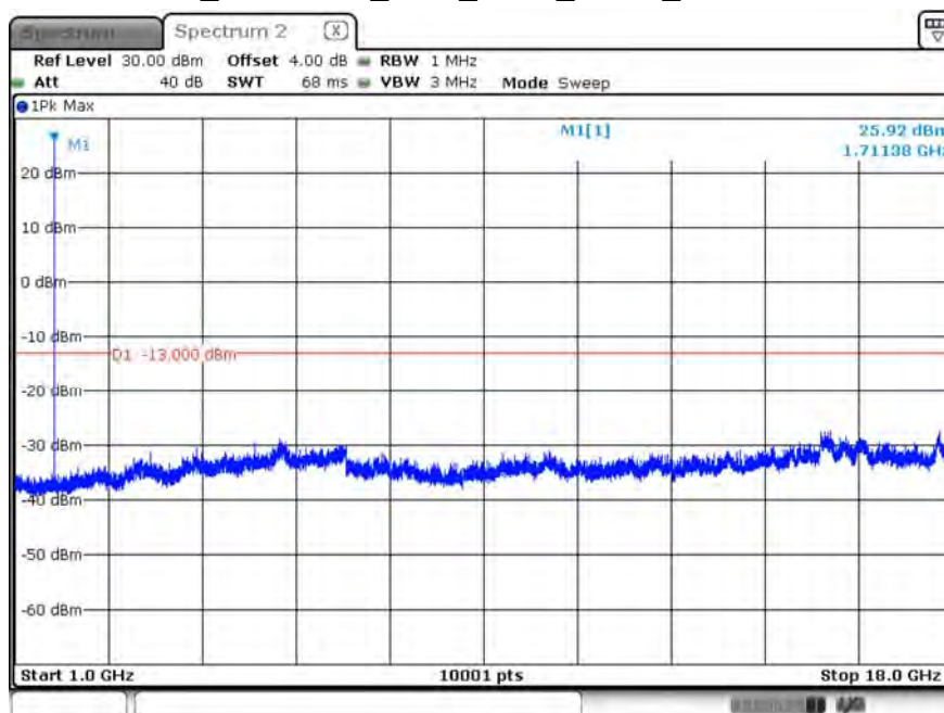
B66_CH131979_1.4M_1RB2_QPSK_Above 1G
