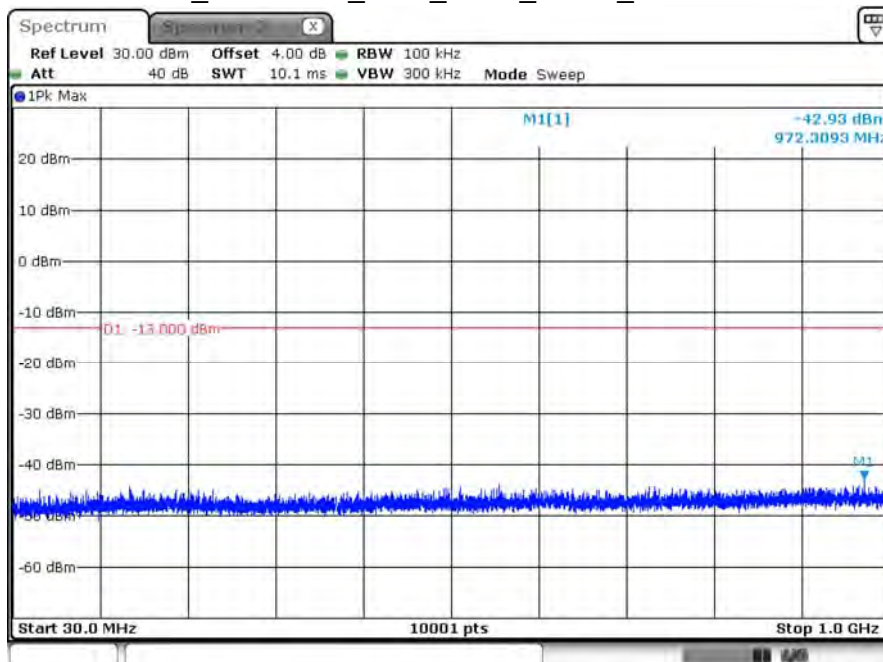
B66_CH132322_1.4M_1RB2_QPSK_Below 1G
