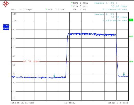
GFSK-Hopping AV-H
