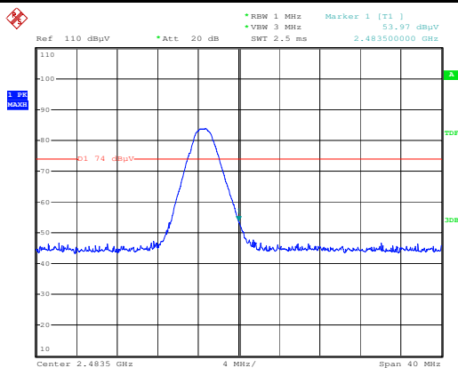
\pi /4DQPSK-Right Side-AV-V
