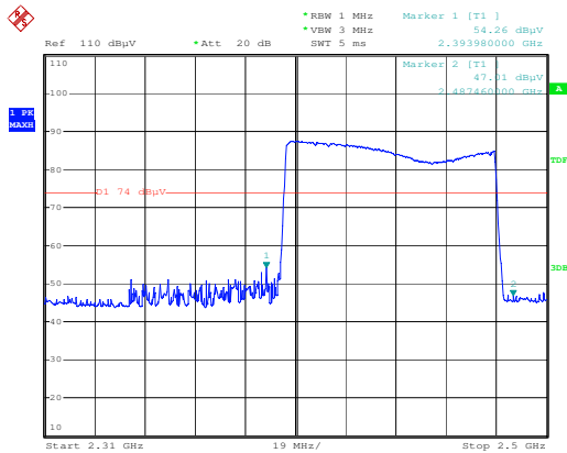
GFSK-Hopping AV-V
