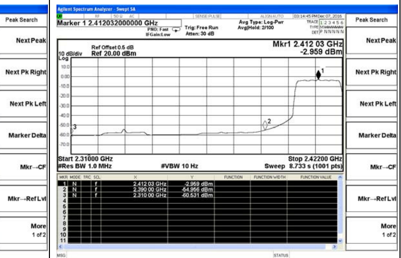
802.11n(HT20)-Low channel(Average)
