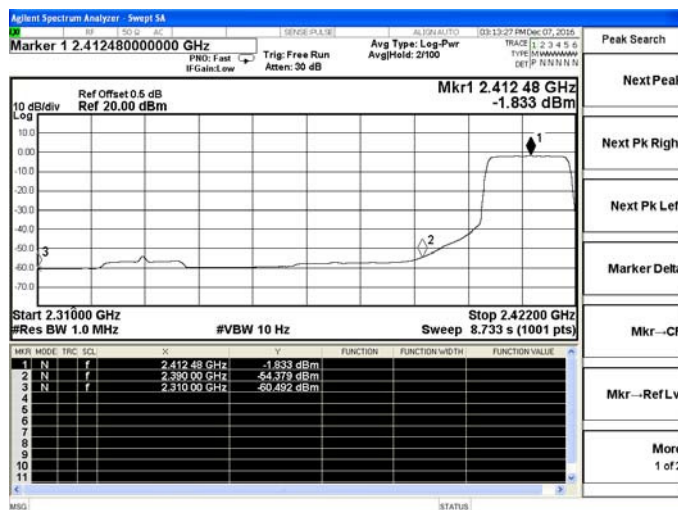
802.11g-Low channel(Average)
