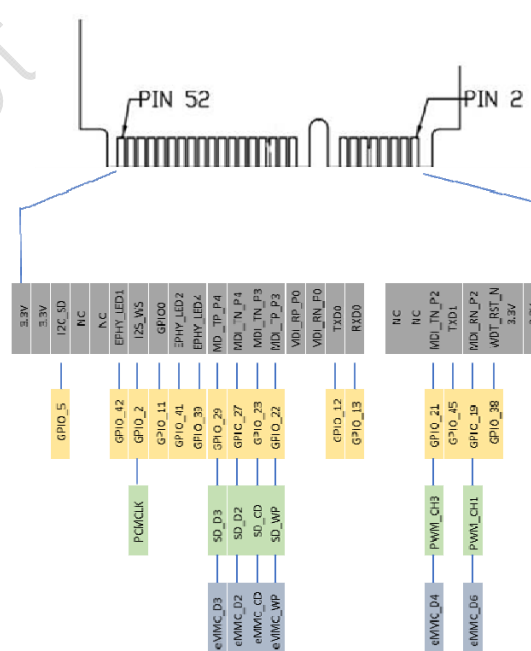
mini PCIe connector Bottom View
