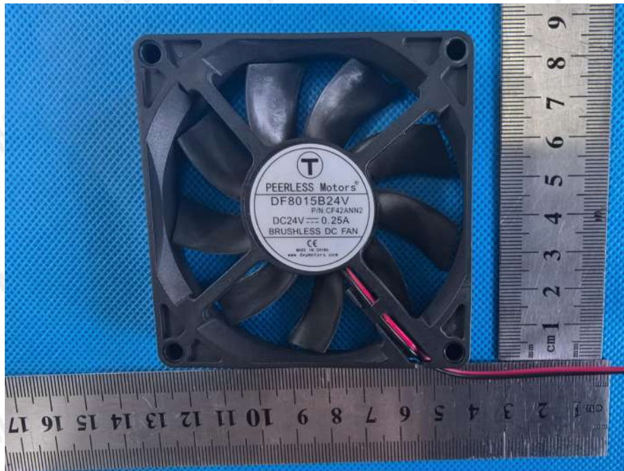
DF8015B24V-CF42ANN2
