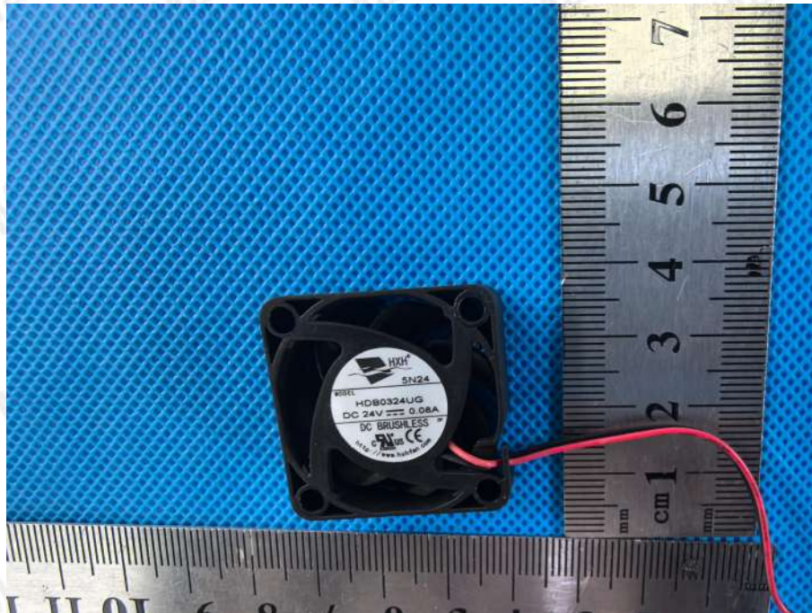
HDB0324UG
