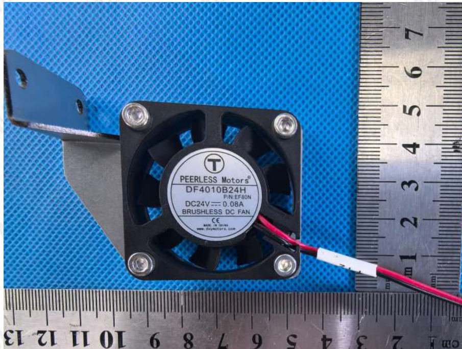
DF4010B24H-EF80N
