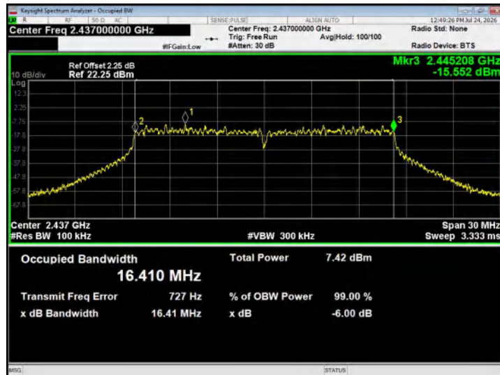
802.11n20 - CH06
