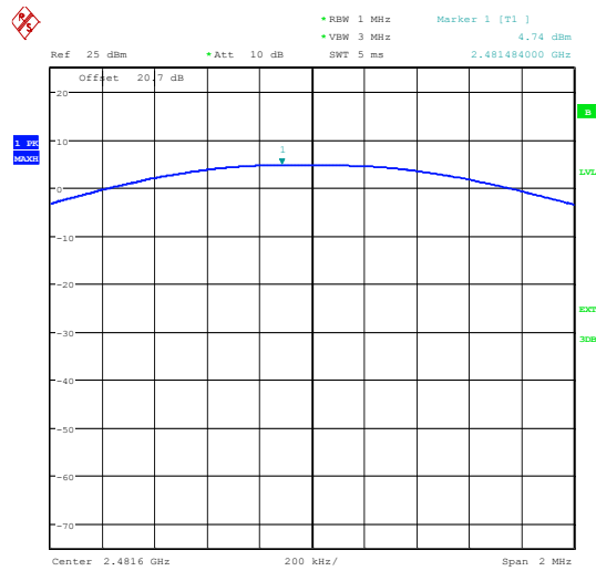
2481.6 MHz
