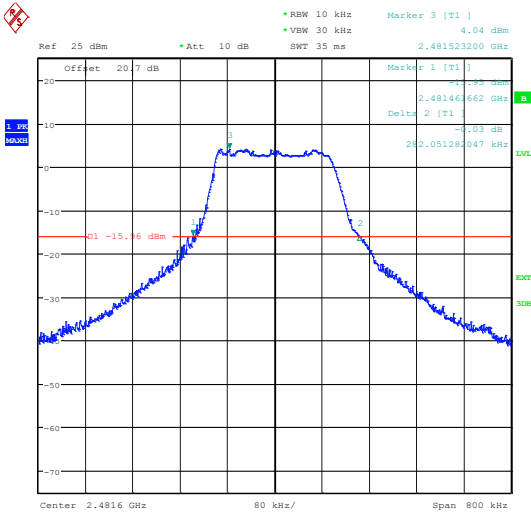
2481.6 MHz
