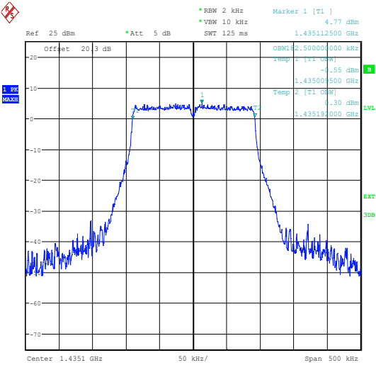
1435.1 MHz
