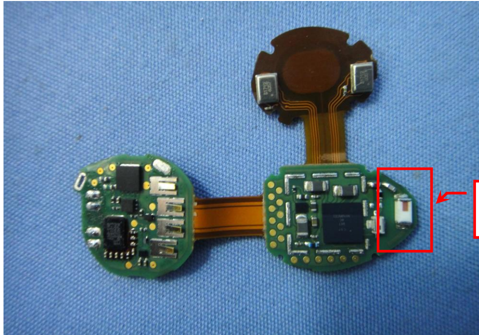
EUT Photo 11 )
