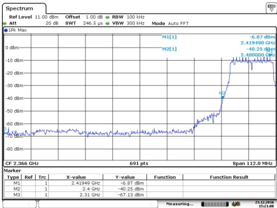
CH01-Bandedge
