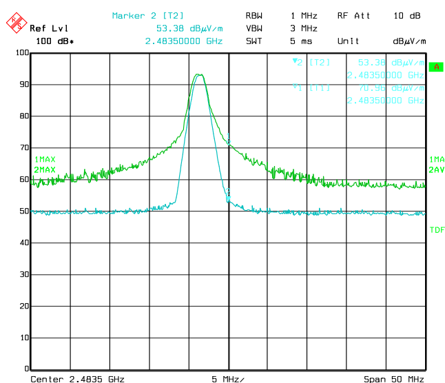
UPPER EDGE
