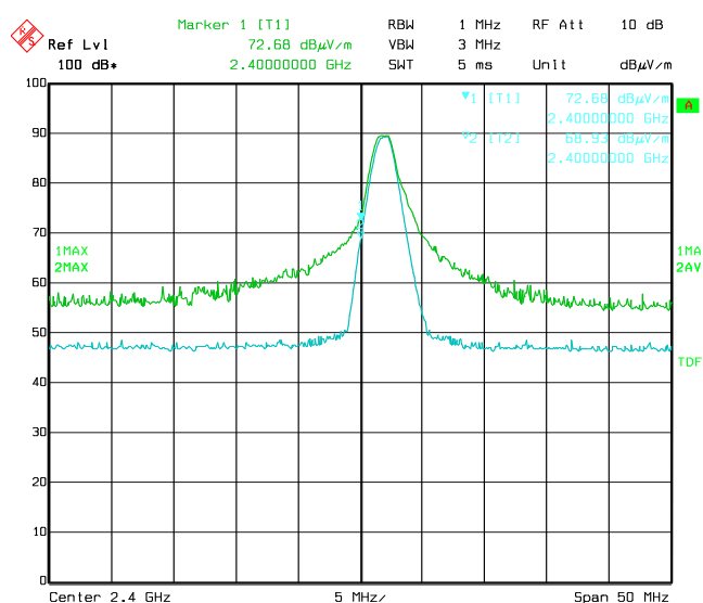
LOWER EDGE
