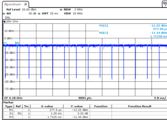
ANT 1
