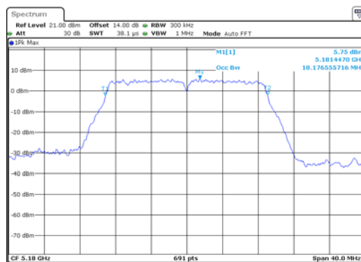
ANT 2(11AC20)
