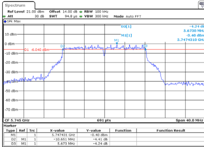
ANT 1(802.11A)
