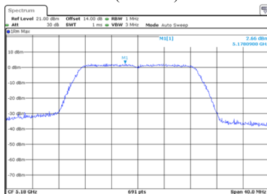
ANT 2(11AC20)
