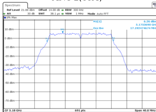
ANT 2(11A)
