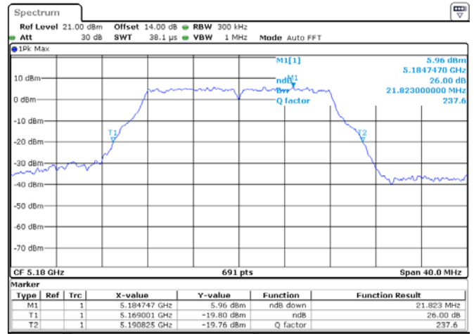
ANT 2(11A)
