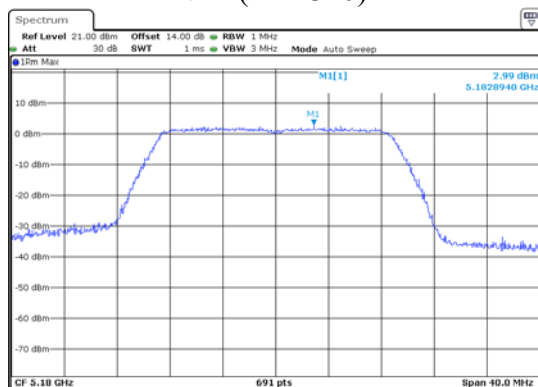
ANT 1(11AC20)
