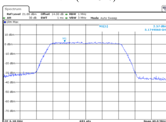
ANT 2(11AC20)
