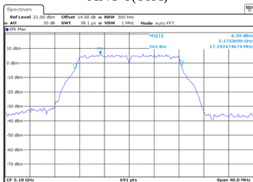
ANT 1(11A)
