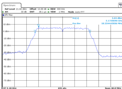
ANT 1(11AC20)
