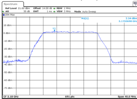
ANT 1(11A)
