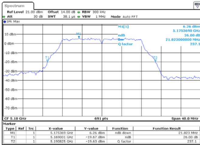
ANT 1(11A)
