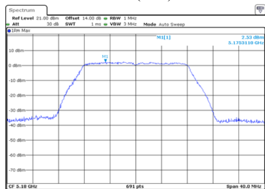
ANT 2(11A)
