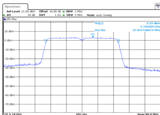
ANT 1(11N40)
