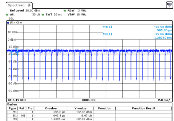
ANT 2
