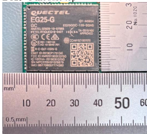
EG25-G module top
