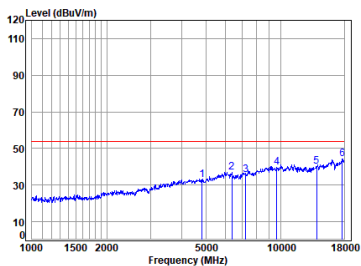
11g_TX_CH_01_Vertical-Avg
