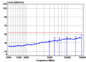
11g_TX_CH_11_Vertical-Avg
