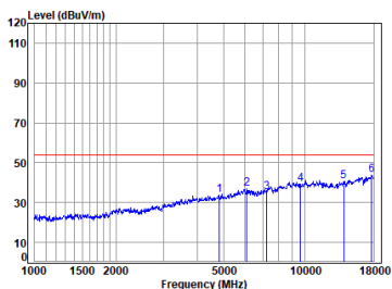
11g_TX_CH_01_Horizontal-Avg
