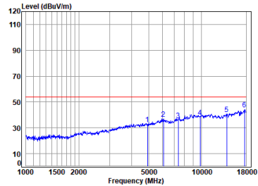
11g_TX_CH_11_Horizontal-Avg
