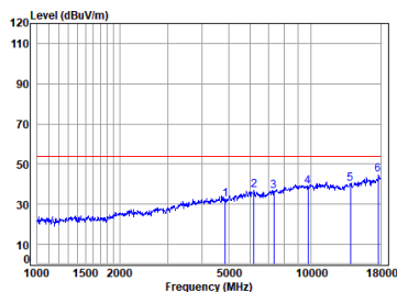
11g_TX_CH_06_Vertical-Avg
