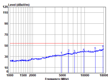
11g_TX_CH_06_Horizontal-Avg
