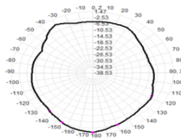
Total(E1-XZ)
