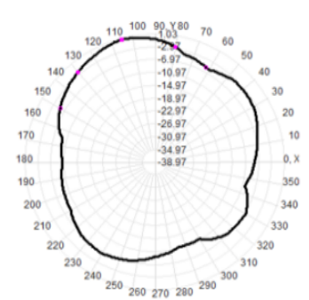
Total(H-XY)
