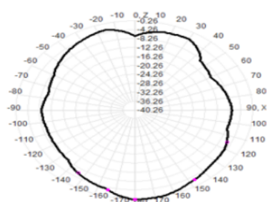
Total(E1-XZ)
