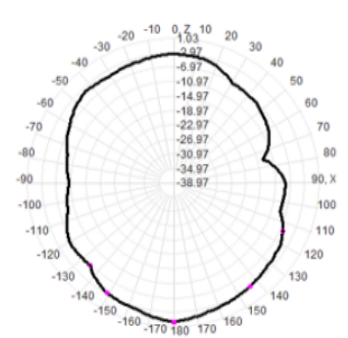
Total(E1-XZ)
