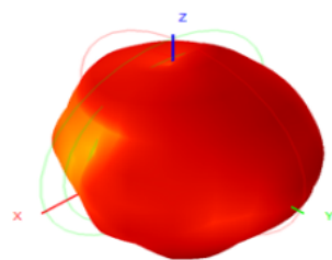
Total(E2-YZ)
