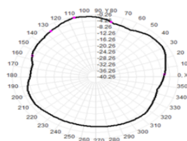
Total(H-XY)
