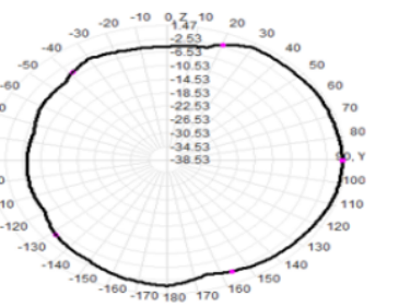
Total(E2-YZ)
