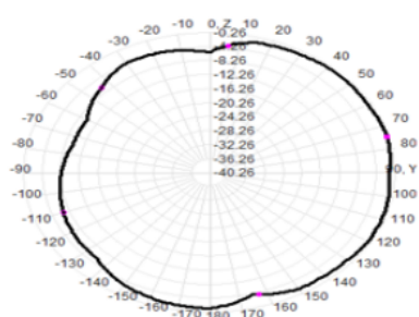
Total(E2-YZ)
