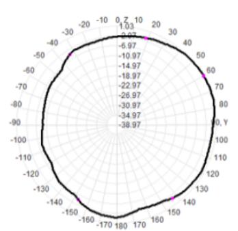
Total(E2-YZ)
