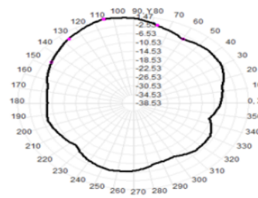
Total(H-XY)
