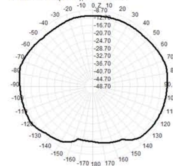
2110.0MHz Total(E2-YZ), Max= -8.70dBi
