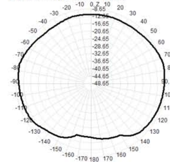
2100.0MHz Total(E2-YZ), Max= -8.65dBi
