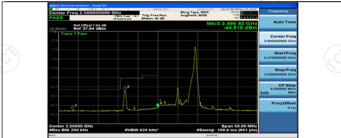
Band7-10MHz-QPSK-20800-25RB#25
