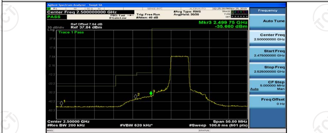
Band7-10MHz-QPSK-20800-25RB#0
