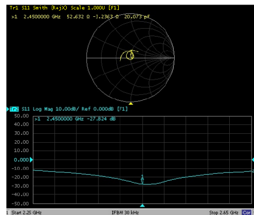
2450MHz Body
