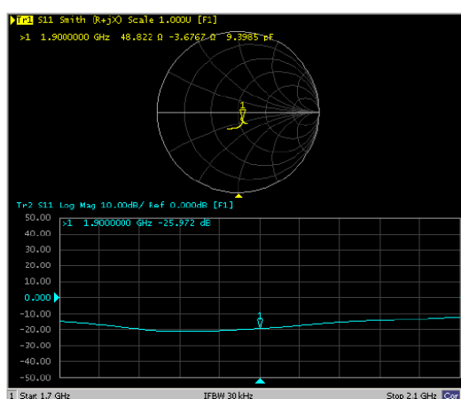
1900MHz Body
