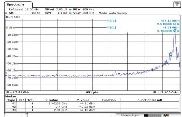
CH00-Bandedge
