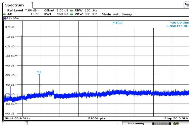
CH39-SE
