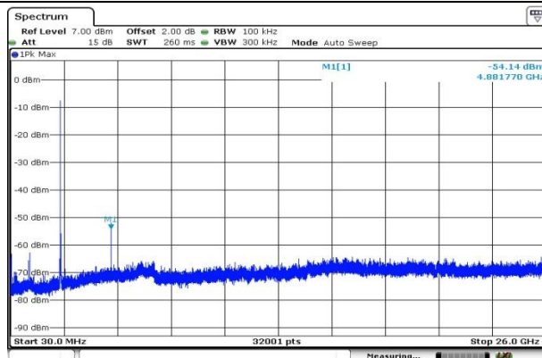
CH19-SE
