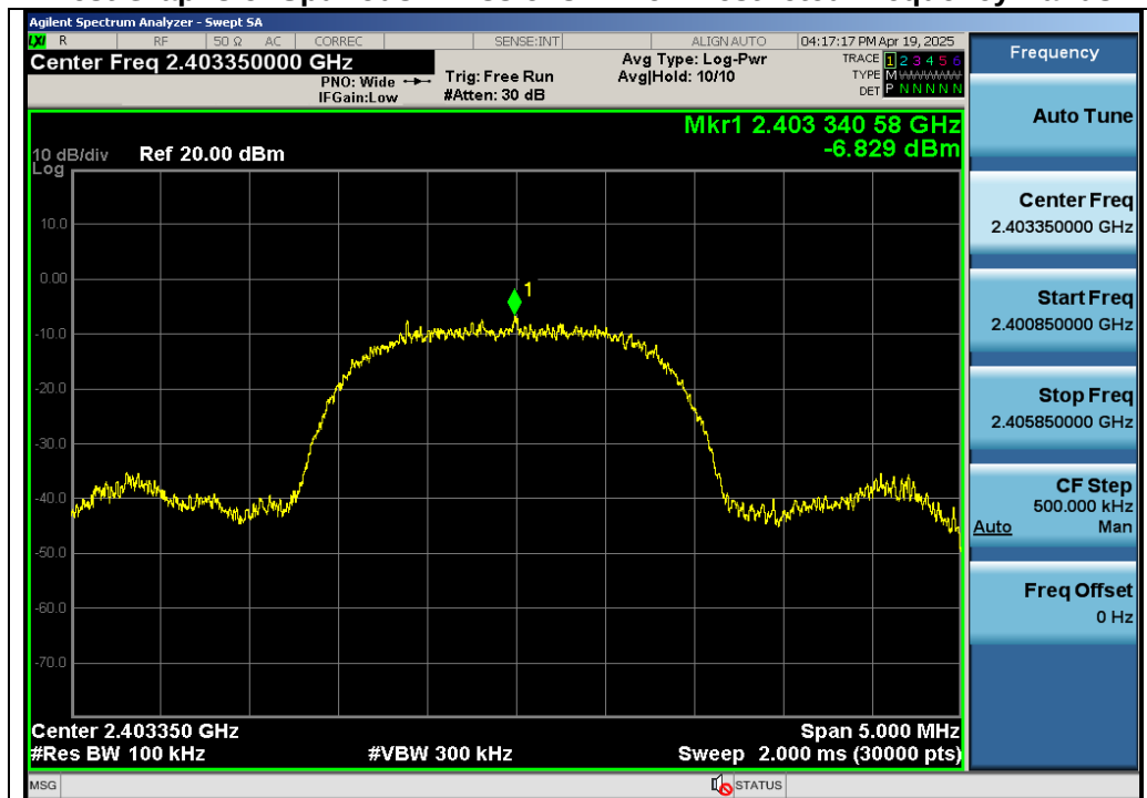
Test_Graph_SRD 2.4G_ANT0_2403.35_Reference Level
