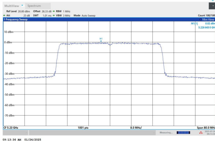
11AX40SISO_Ant1_5230
