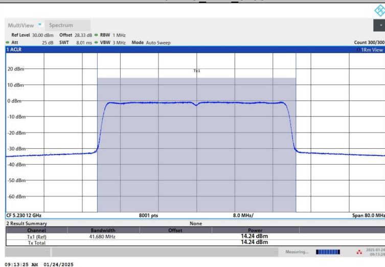
11AX40SISO_Ant1_5230
