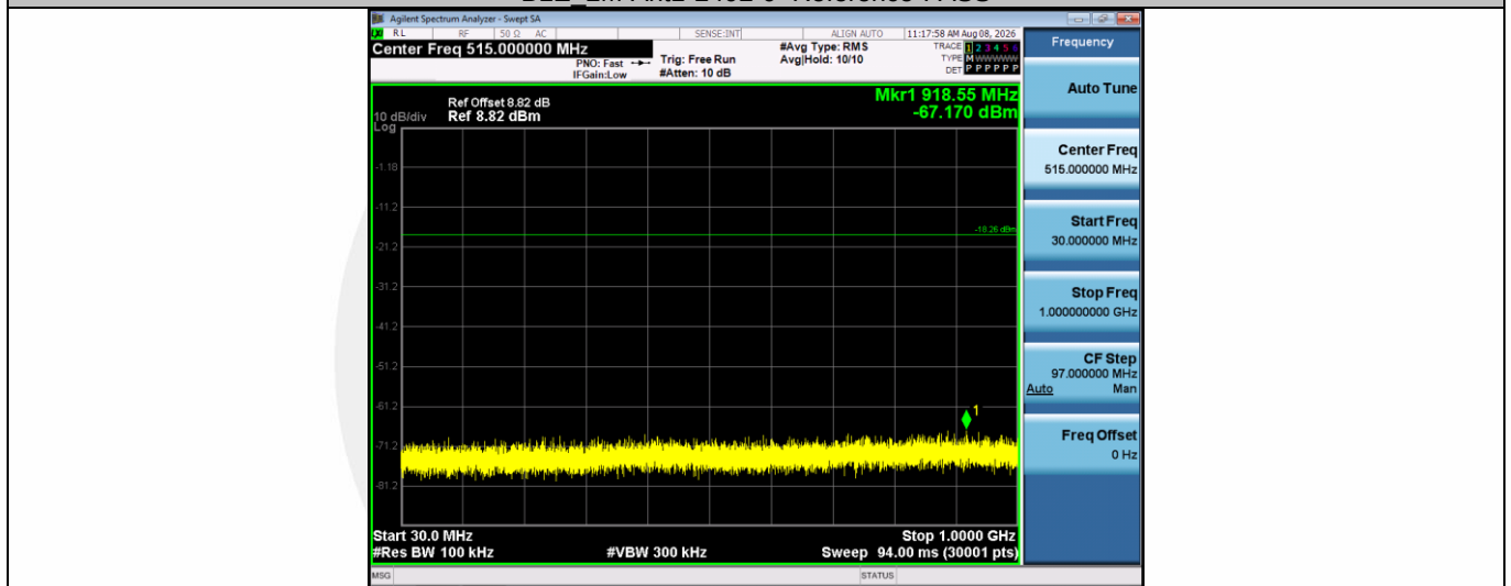
BLE 2M-Ant1-2402-30~1000-PASS
