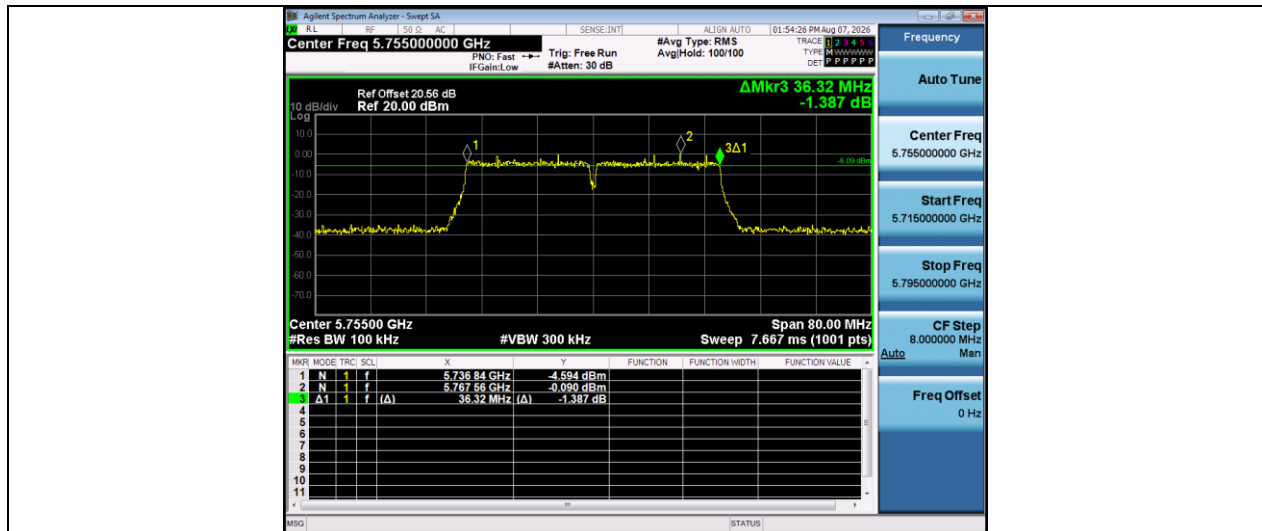
11N40SISO-Ant1-5755-PASS
