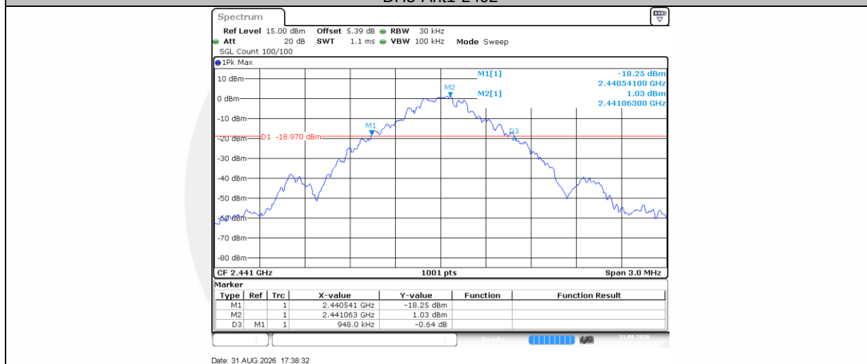
DH5-Ant1-2441
