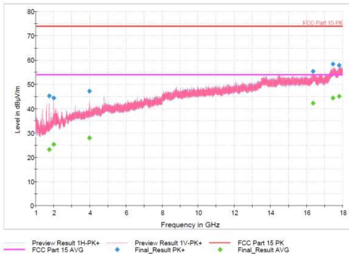
Plot 25. 1-18GHz, 2440MHz
