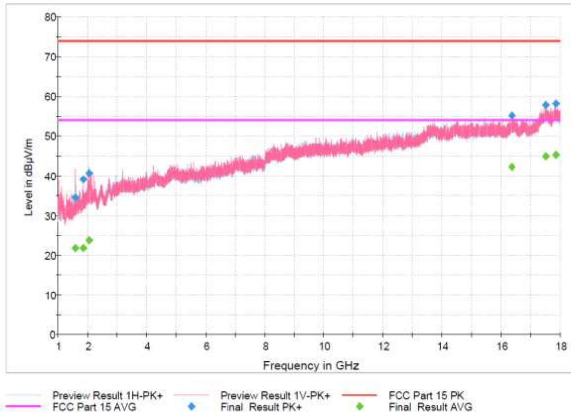
Plot 24. 1-18GHz, 2402MHz
