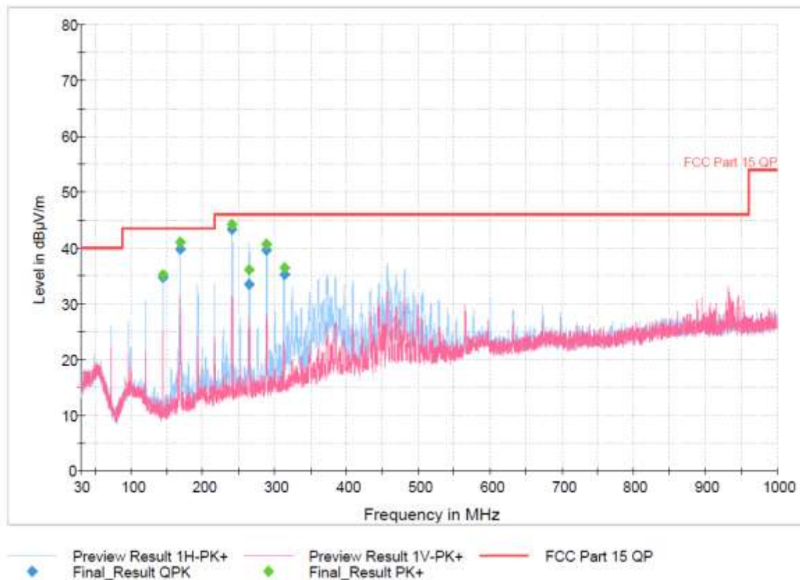
Plot 22. 30MHz-1000MHz, 2440MHz
