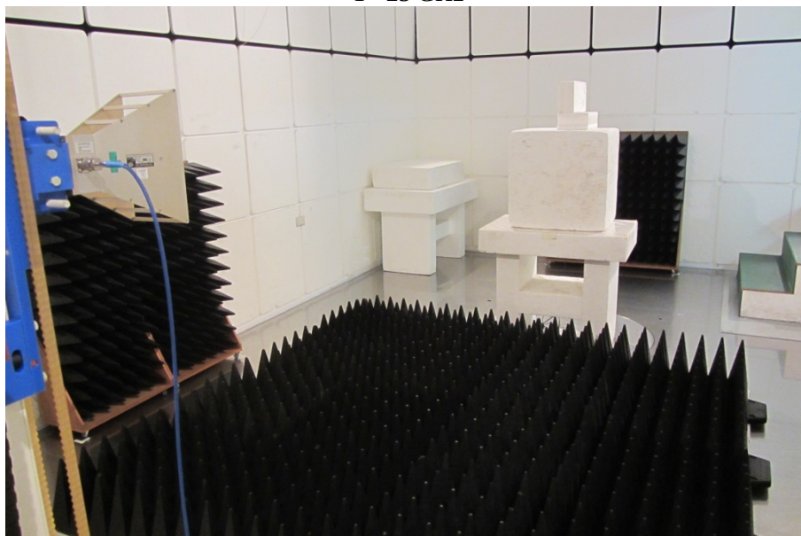
1 - 25 GHz
