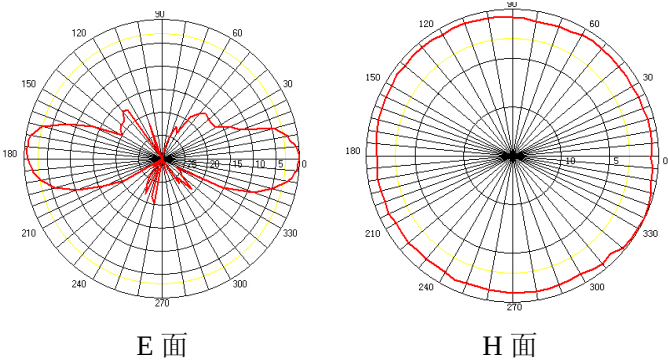
参考方向图
