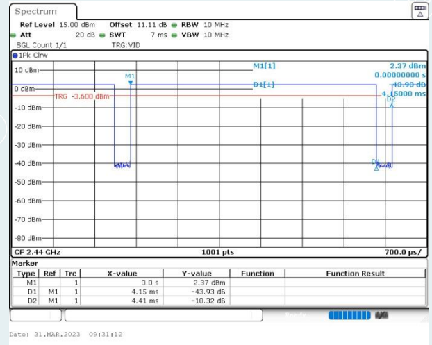
Zigbee_2440MHz
