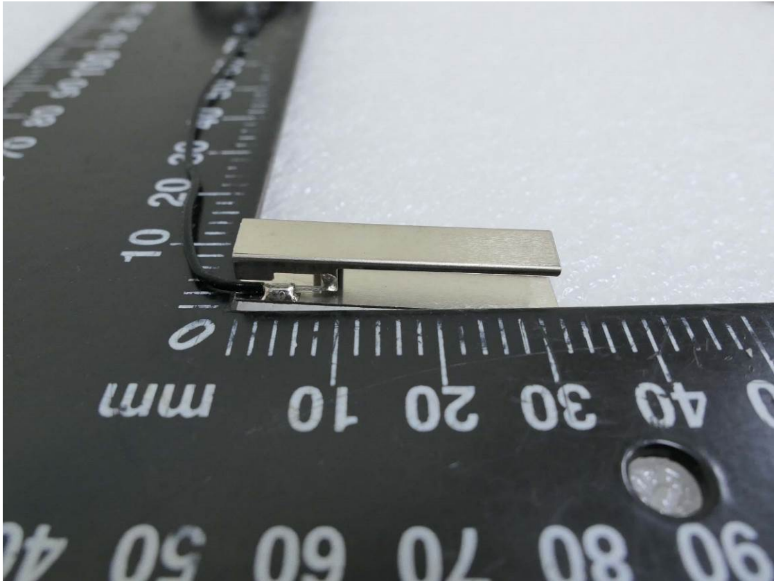
EUT-21. Antenna
