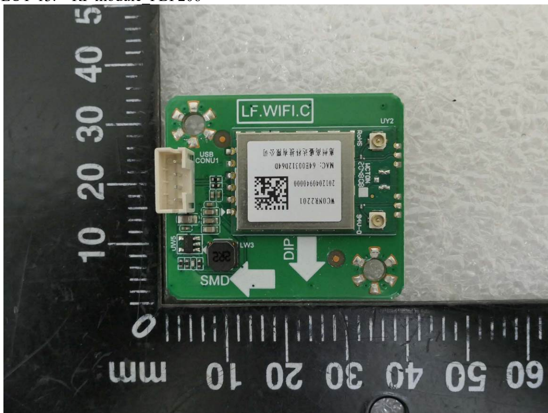
EUT-13. RF module FBP206
