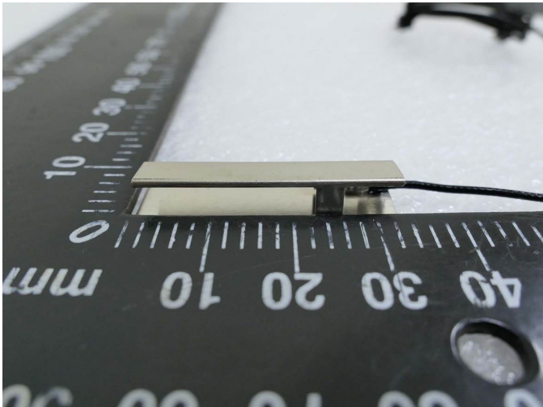
EUT-20. Antenna
