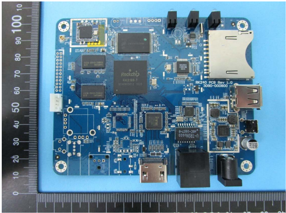
(2) Module Photo
