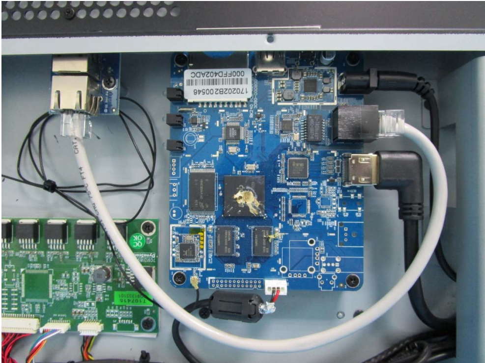
(2) Module Photo
