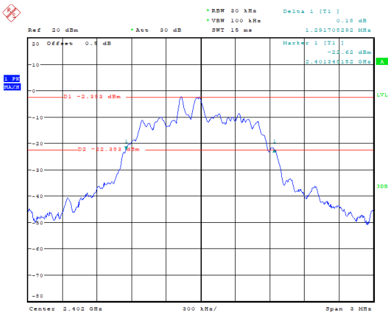
\pi/4 -DQPSK_Low 1.292 MHz
