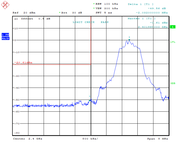
\pi/4 -DQPSK_Low 49.56 dB
