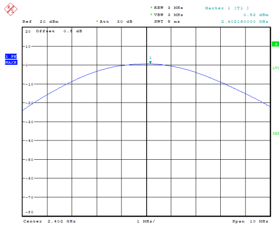
\pi/4 -DQPSK_Low 0.52 dBm
