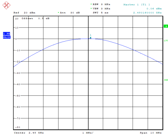
\pi/4 -DQPSK_High 0.06 dBm
