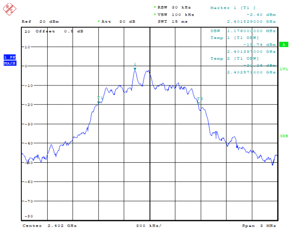
\pi/4 -DQPSK_Low 1.176 MHz
