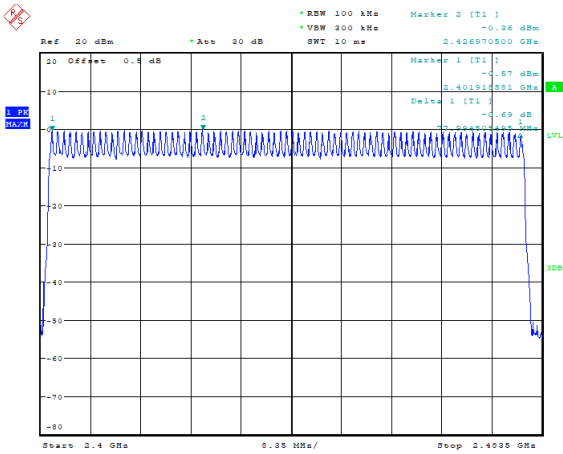
\pi/4 -DQPSK_Hopping 79
