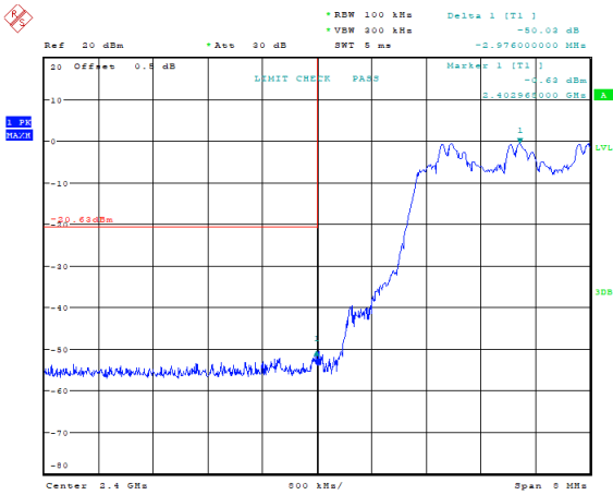
\pi/4 -DQPSK_Hopping_Lower 50.03 dB
