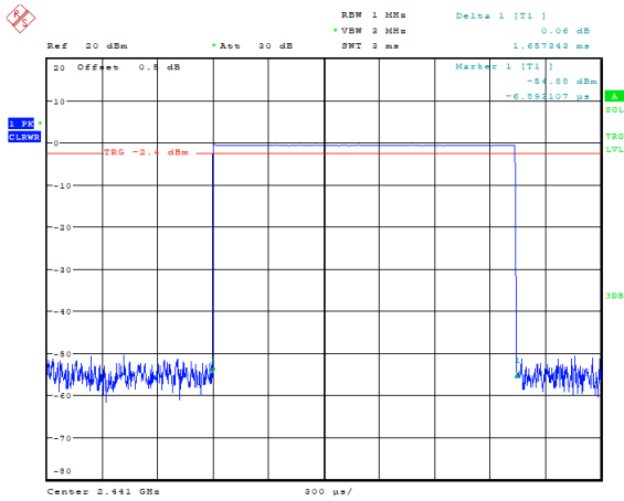
GFSK_Hopping_DH3 1.657ms
