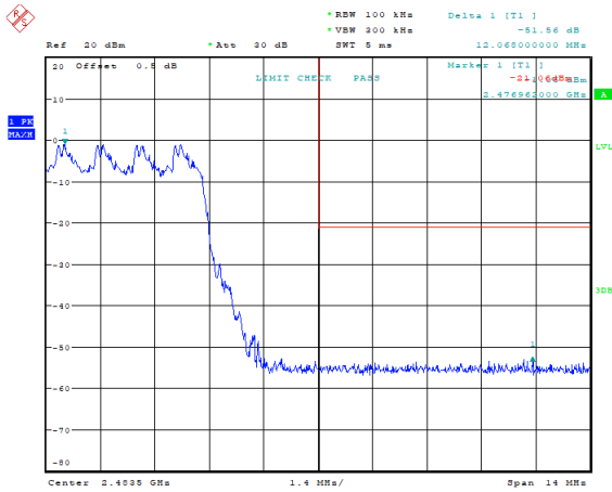
\pi/4 -DQPSK_Hopping_Upper 51.56 dB
