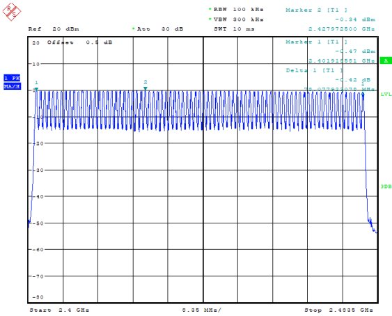
GFSK_Hopping 79
