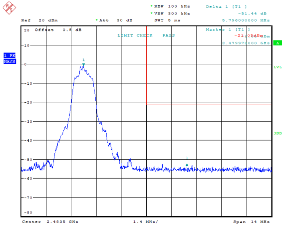
\pi/4 -DQPSK_High 51.44 dB
