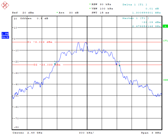
\pi/4 -DQPSK_High 1.301 MHz
