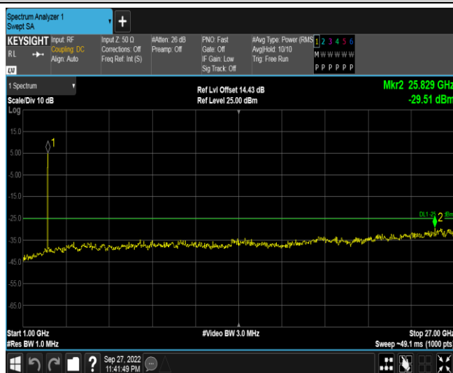
Band41-10MHz-QPSK-39700-1RB#0-Range2:1000~27000MHz
