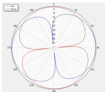
Theta=0 freq=2500MHz
