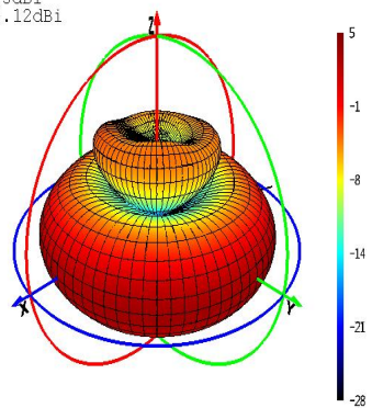
Theta=0 freq=2500MHz
