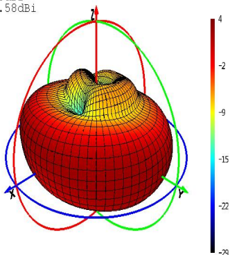
Theta=0 freq=2500MHz
