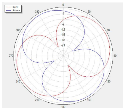
Theta=0 freq=2500MHz
