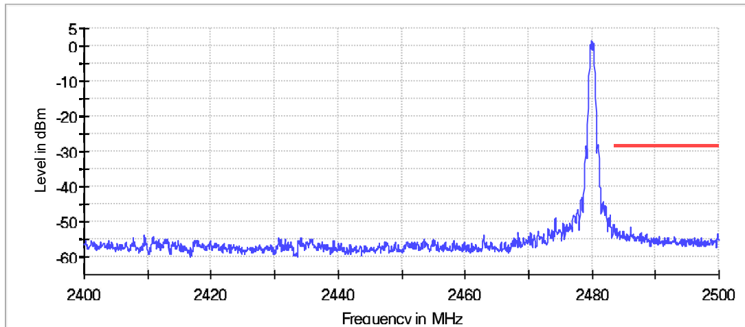
Band Edge
