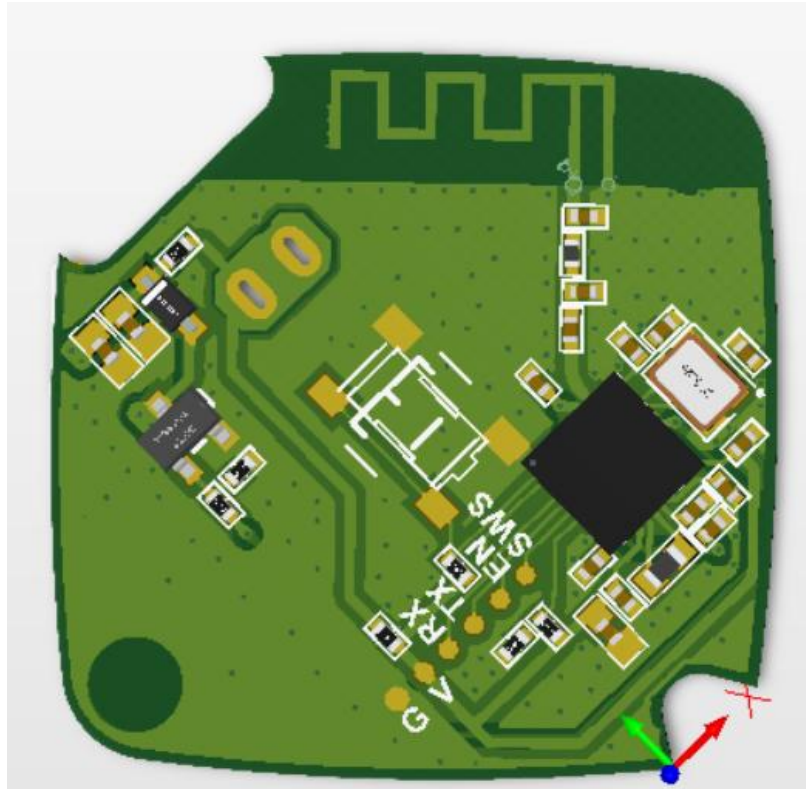
GTAG WiFi Module
